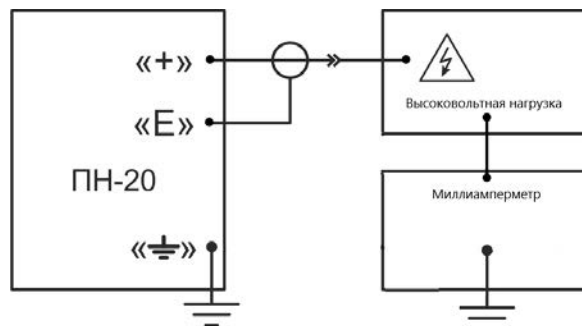
Рисунок 2 – Схема соединения при измерении силы постоянного электрического тока
