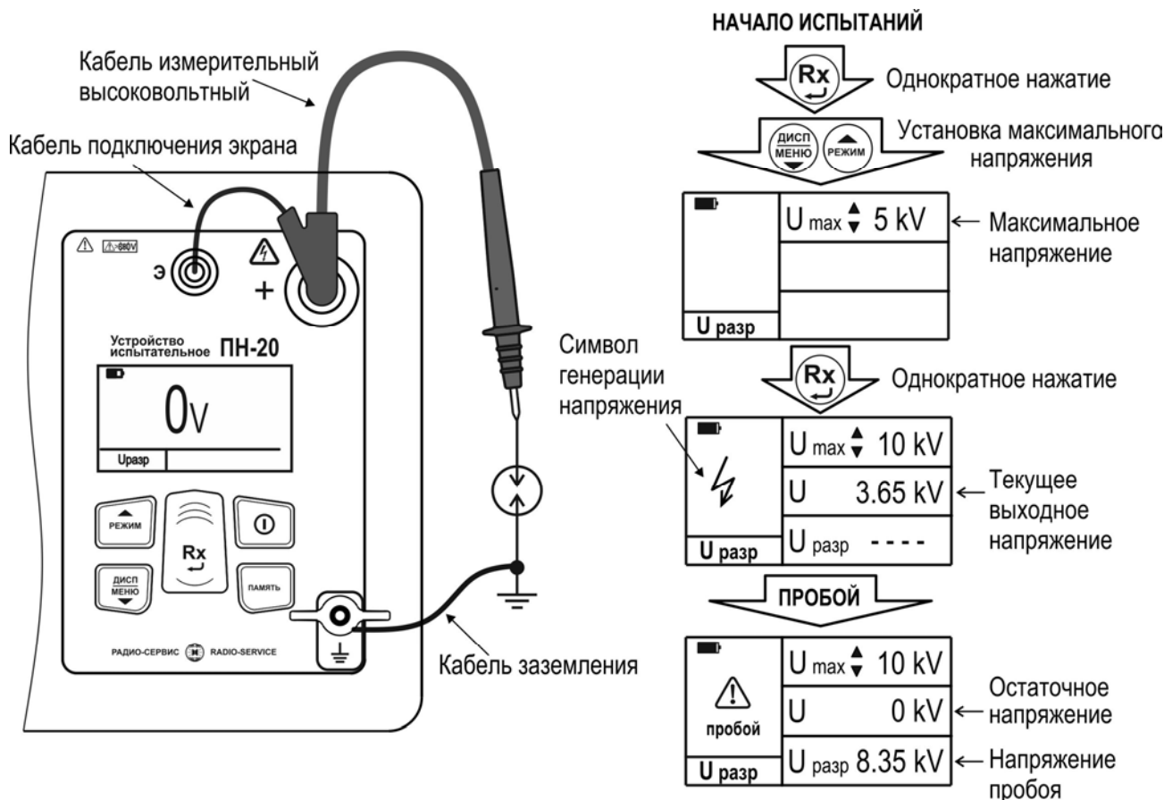
Рисунок 8 - Проверка напряжения пробоя разрядников
