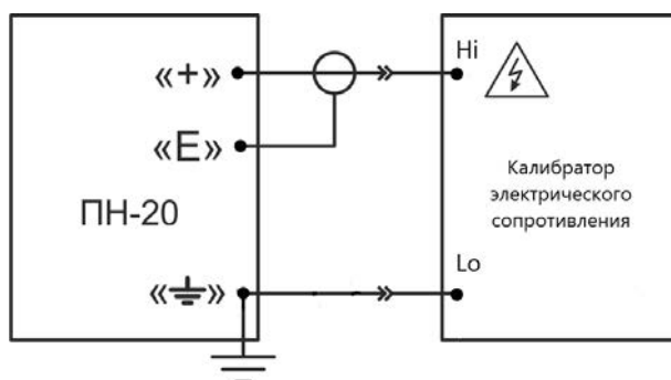
Рисунок 3 – Схема соединения при измерении электрического сопротивления
