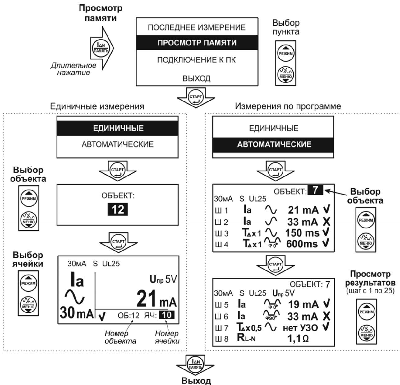
Рисунок 2.46 – Просмотр памяти
